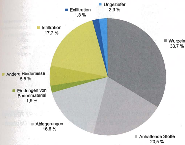
Abb. 9: Schadensverteilung zur betrieblichen Struktur der Kanäle (n = 160; Σ = 67 319 km)
