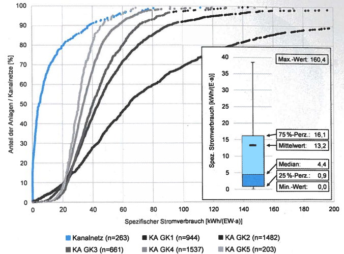
Abb. 6: Spezifischer Stromverbrauch im Kanalnetz in kWh pro Jahr je Einwohner*in (n = 263; Σ = 89 912 km) KA GK = Kläranlage Größenklasse
