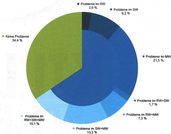
Abb. 16: Probleme und auftretende Orte durch Dränageleitungen ( n = 180 ; \Sigma = 68\,807 km) SW = Schmutzwasser; MW = Mischwasser; RW = Regenwasser
