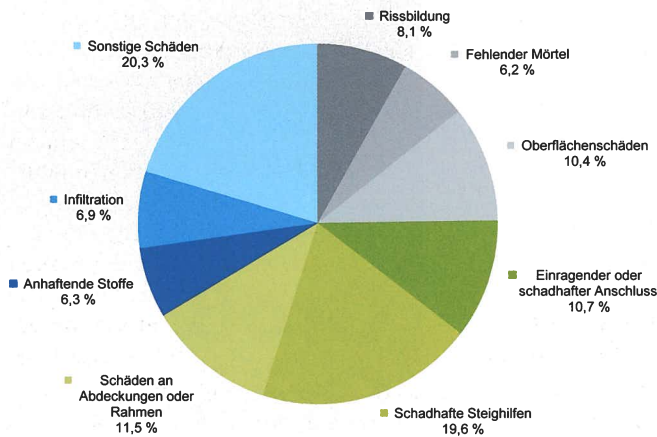
Abb. 11: Schadensverteilung zur baulichen und betrieblichen Struktur der Schächte (n = 113; Σ = 51 073 km)
