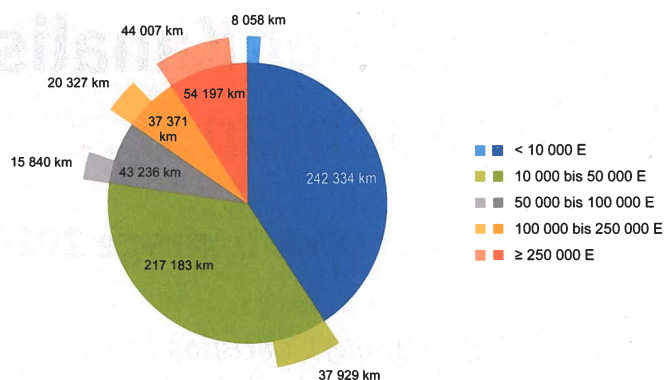
Abb. 1: Gegenüberstellung der in der Umfrage repräsentierten Kanalnetzlängen (n = 423; Σ = 126 161 km) (äußerer Ring) und der gesamten Kanalnetzlänge Deutschlands gemäß Statistischem Bundesamt [9] (innerer Ring)
