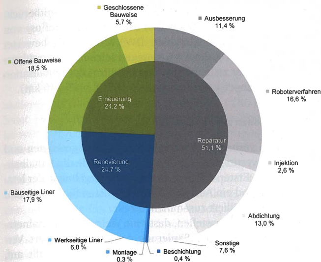
Abb. 14: Verteilung der Sanierungsverfahren (n = 202; Σ = 83 510 km)
